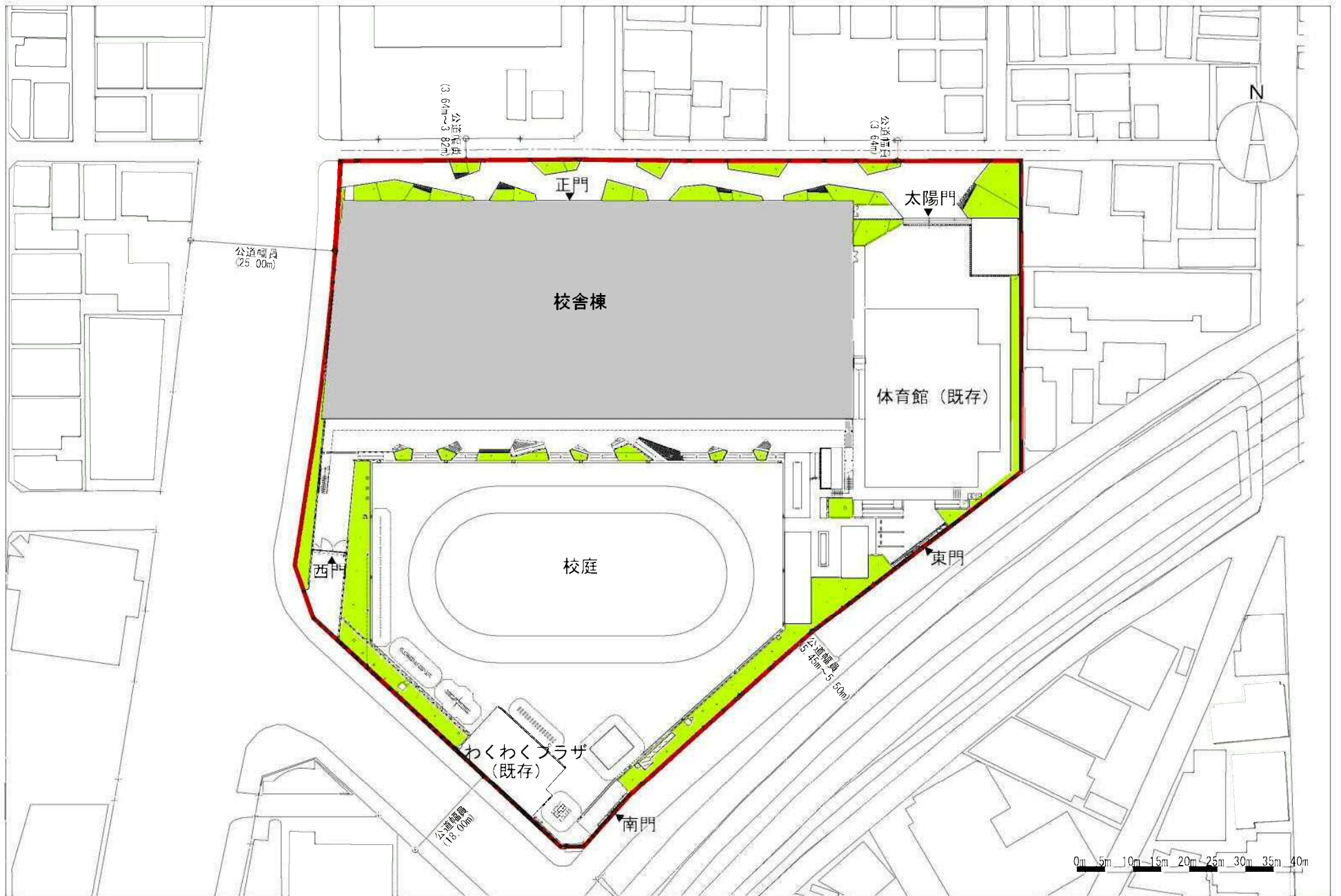
配置図
