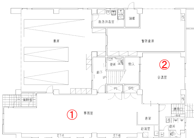
1 階平面図
