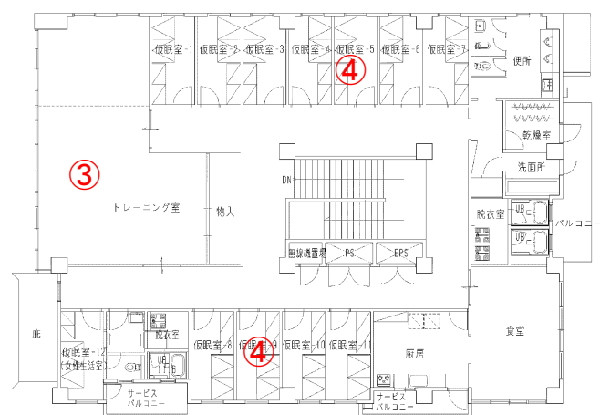
2 階平面図
