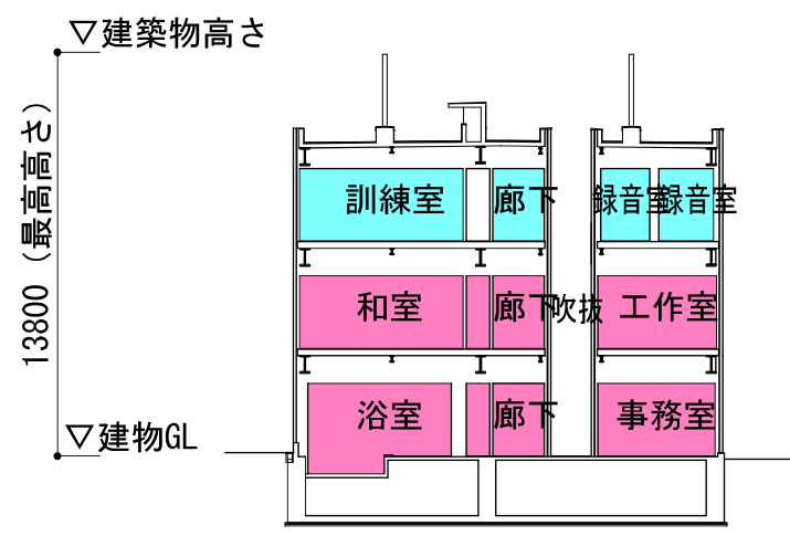
B-B 断面図
