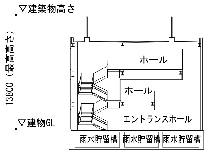
D-D 断面図
