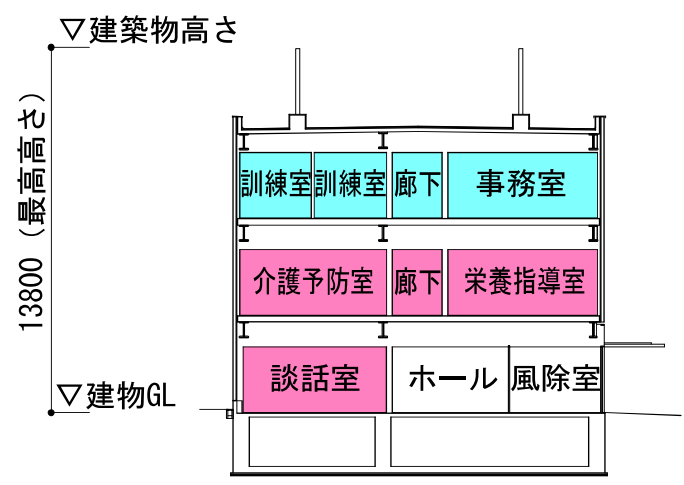
C-C 断面図
