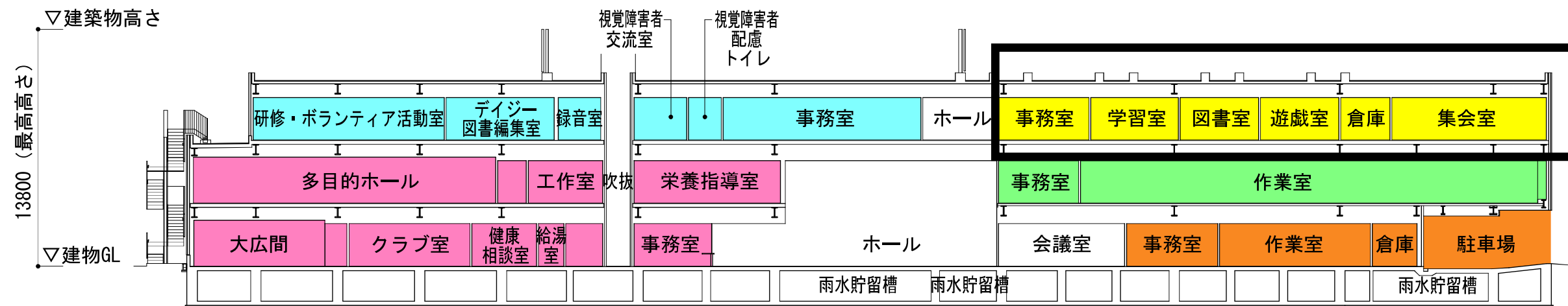
A-A 断面図
