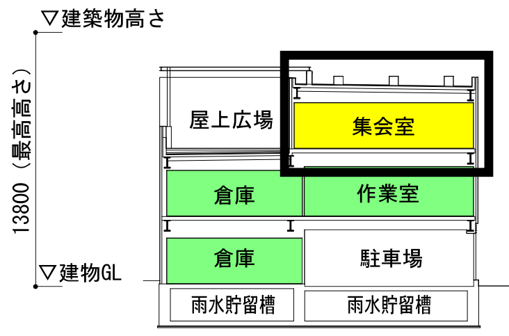
E-E 断面図
