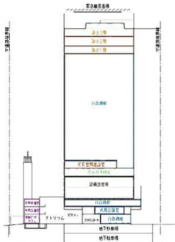
南北断面図
