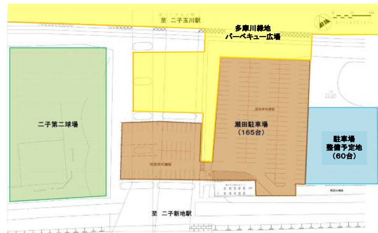
図3 瀬田駐車場平面図
