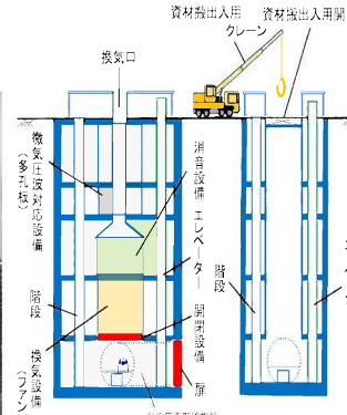
非常口の概要
