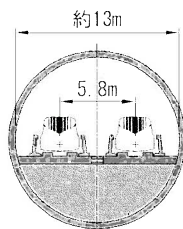
(トンネル)
