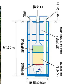
非常口の概要
