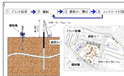
非常口の概要
