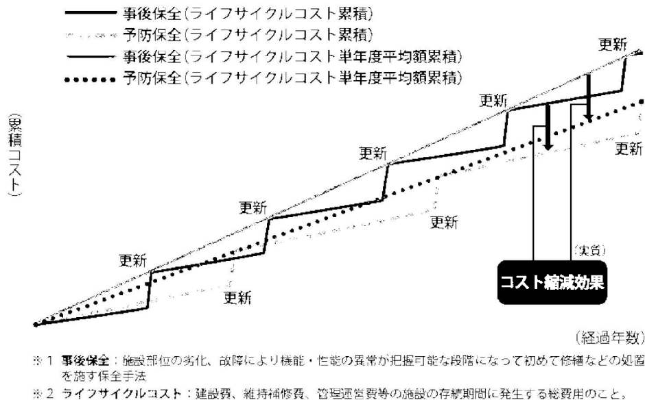
図1 事後保全と予防保全のライフサイクルコスト比較イメージ
