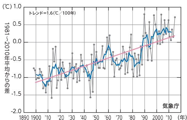
日本の平均気温偏差
