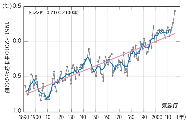
世界の平均気温偏差
