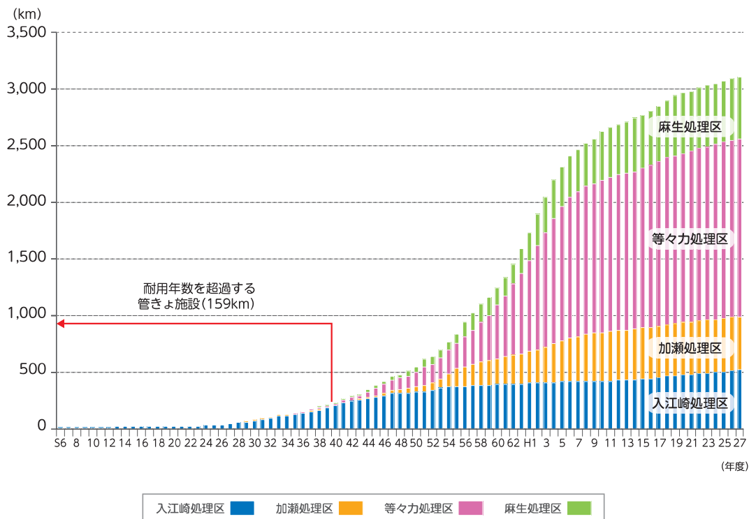
下水道管きよの年度別累計延長の推移(平成27年度末)
