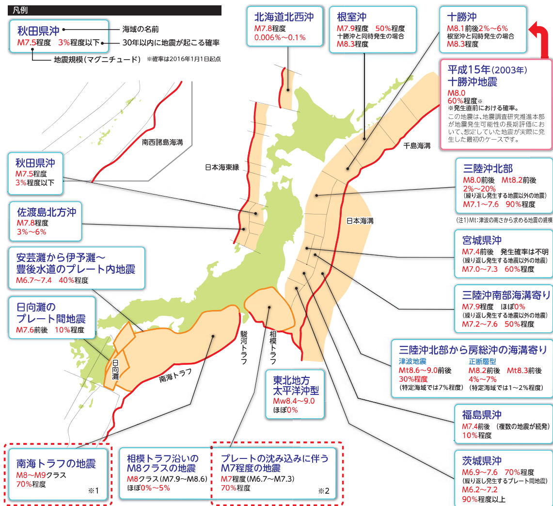
主な海溝型地震の評価結果(2016年1月13日現在)
