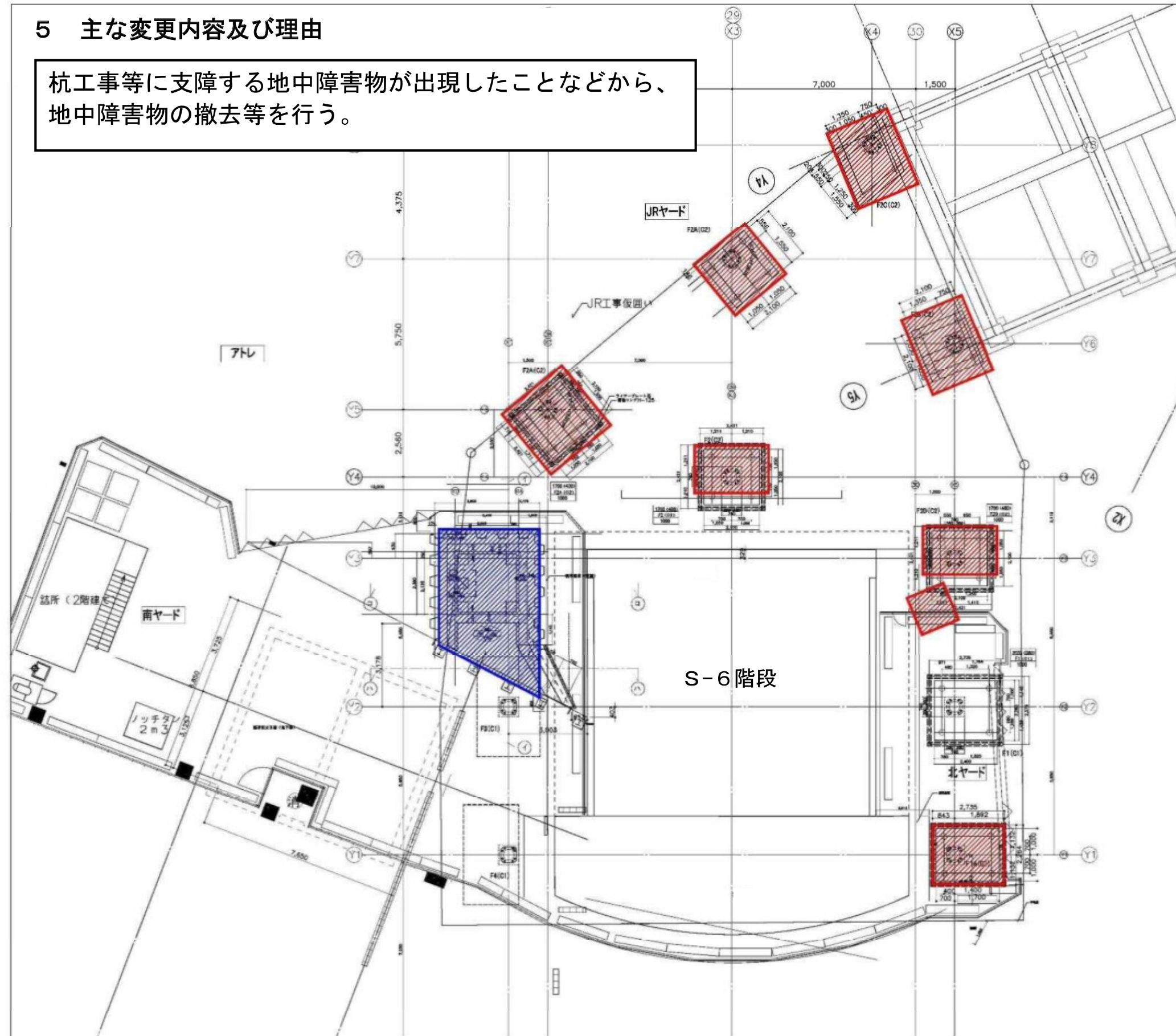
屋根基礎部地中障害物
