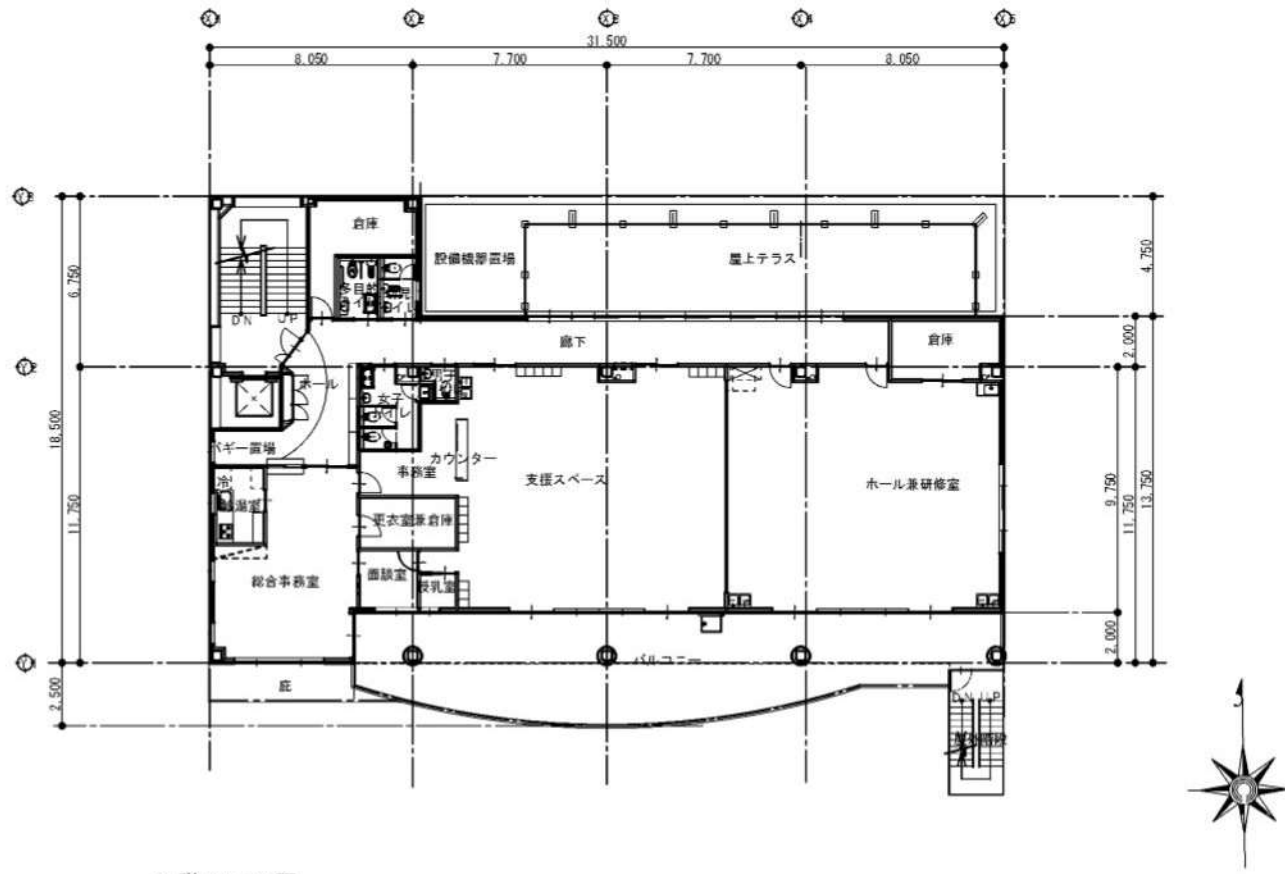
3階平面図
