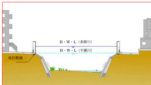
平瀬川の堤防整備
