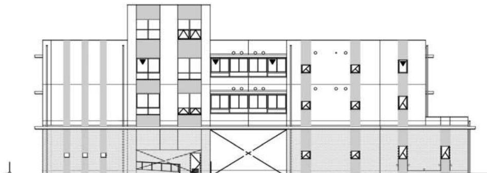
東側立面図
