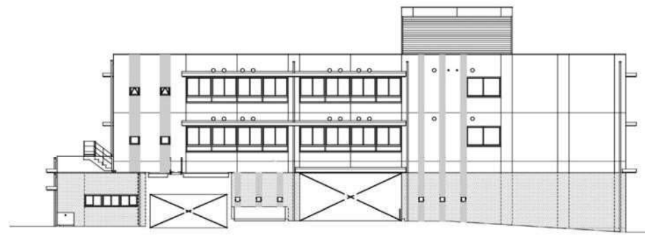
西側立面図
