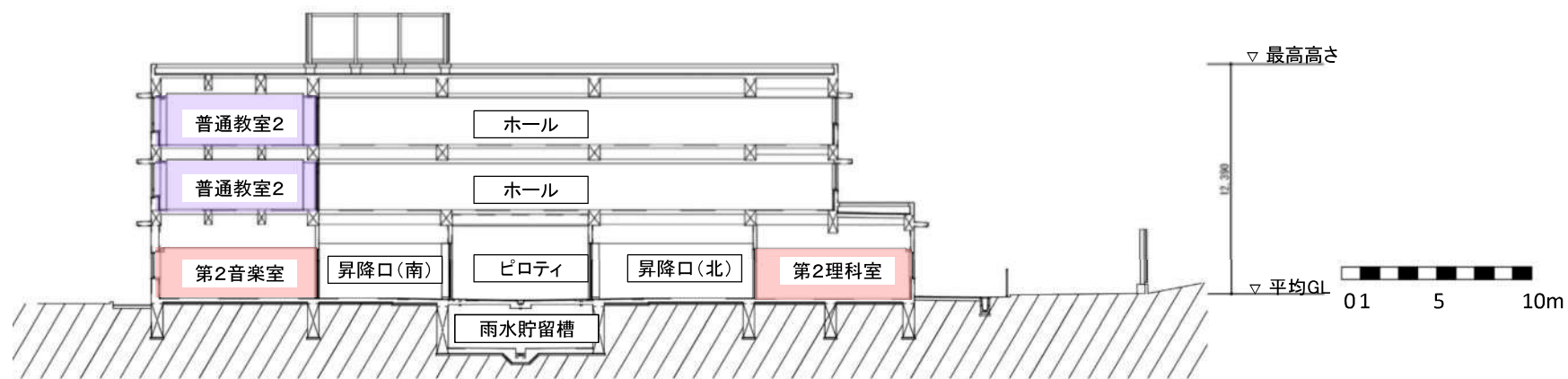
B-B'断面図
