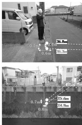
【吐き口部状況写真】
