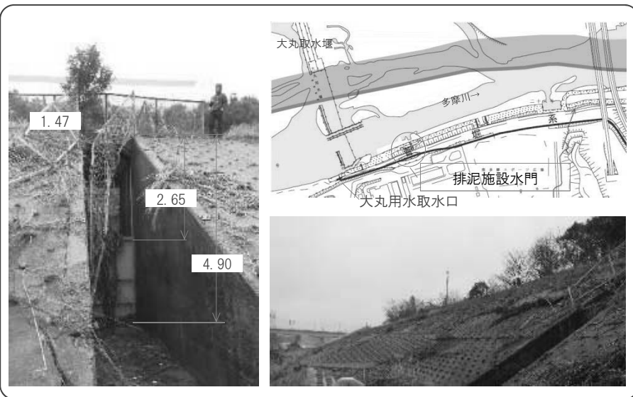
大丸用水排泥施設水門の状況
