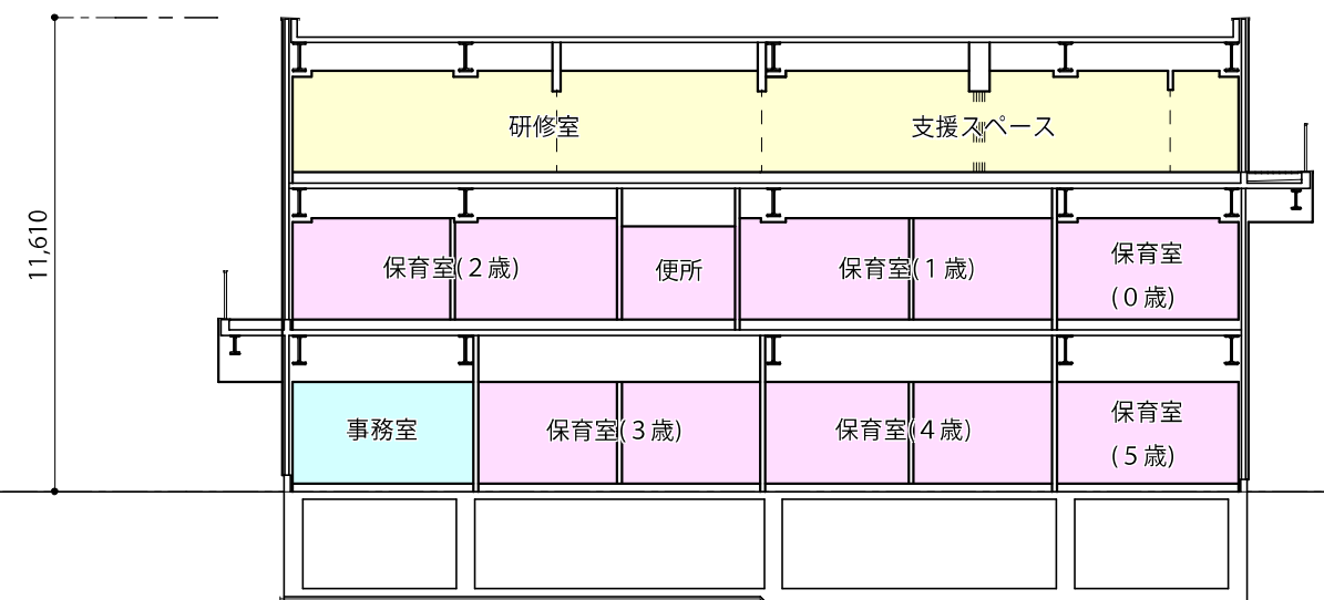
断面図 2
