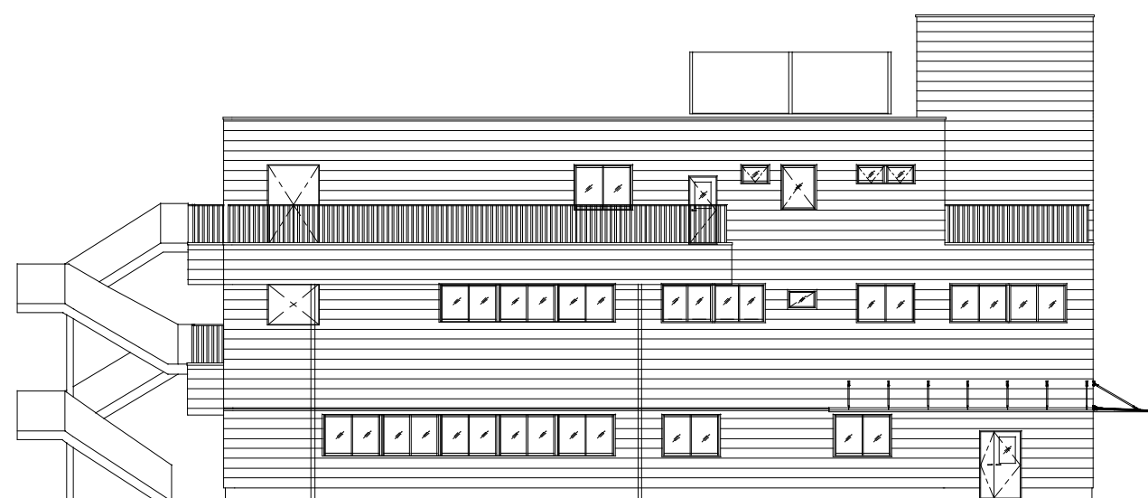
北立面图
