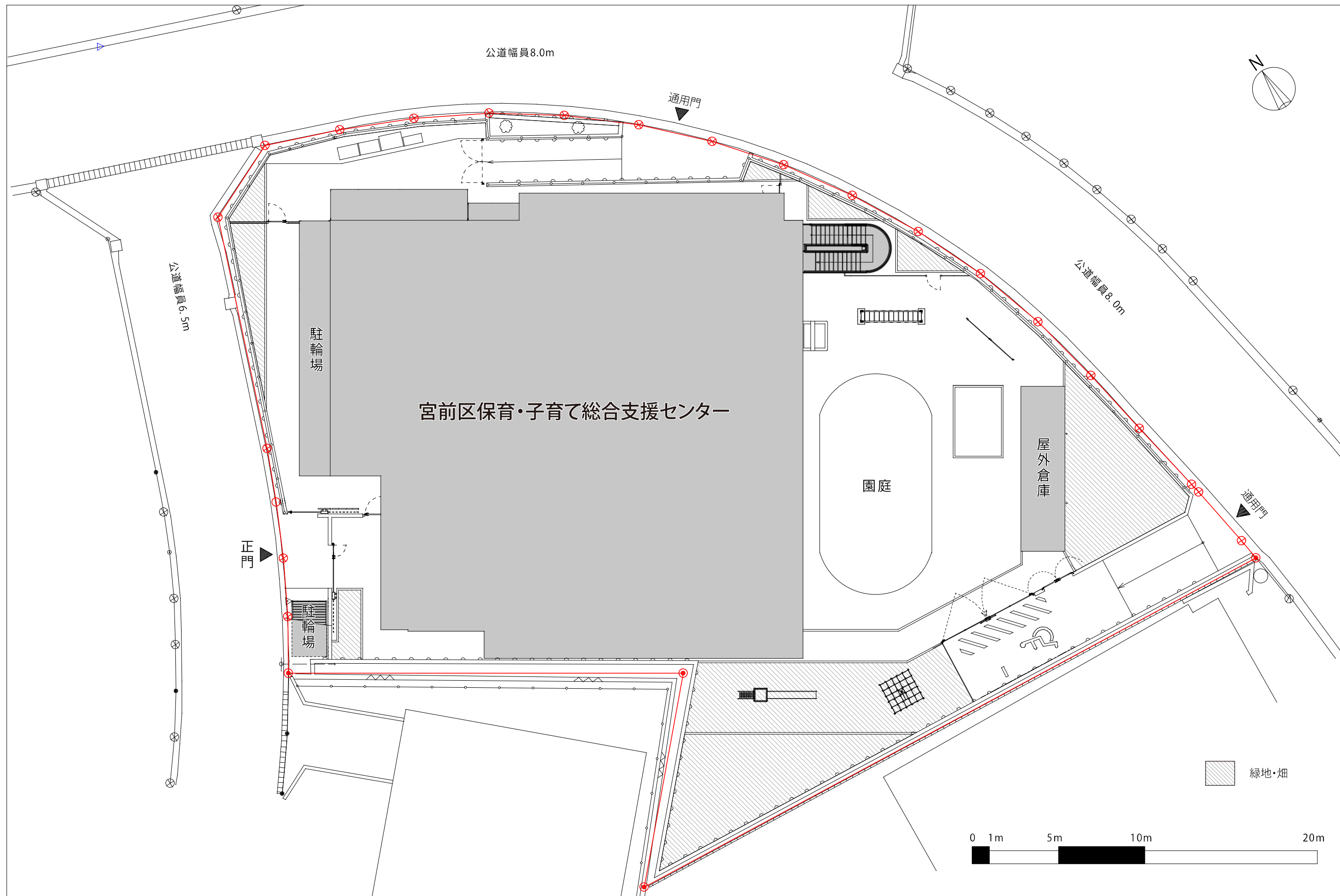
配置図
