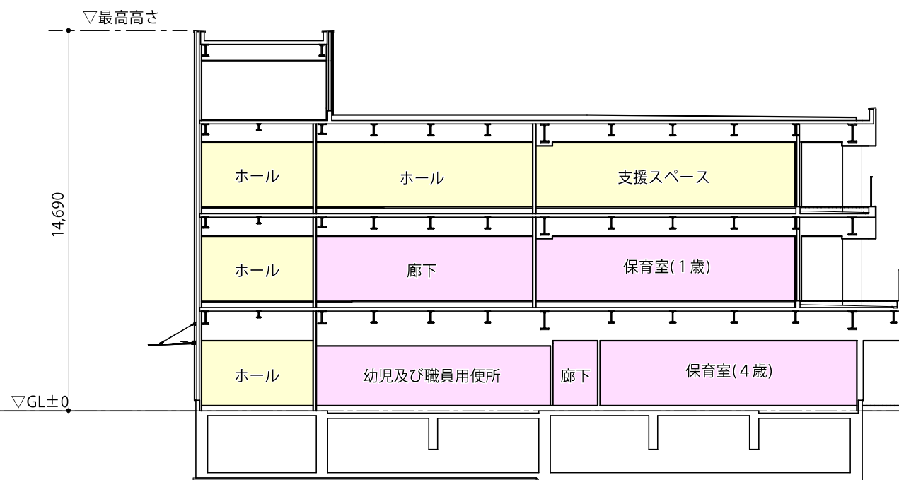
断面図 1
