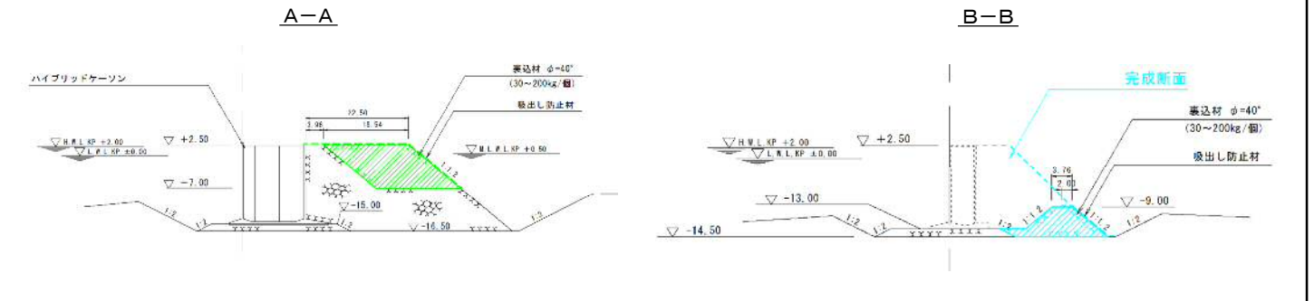
(断面図)
