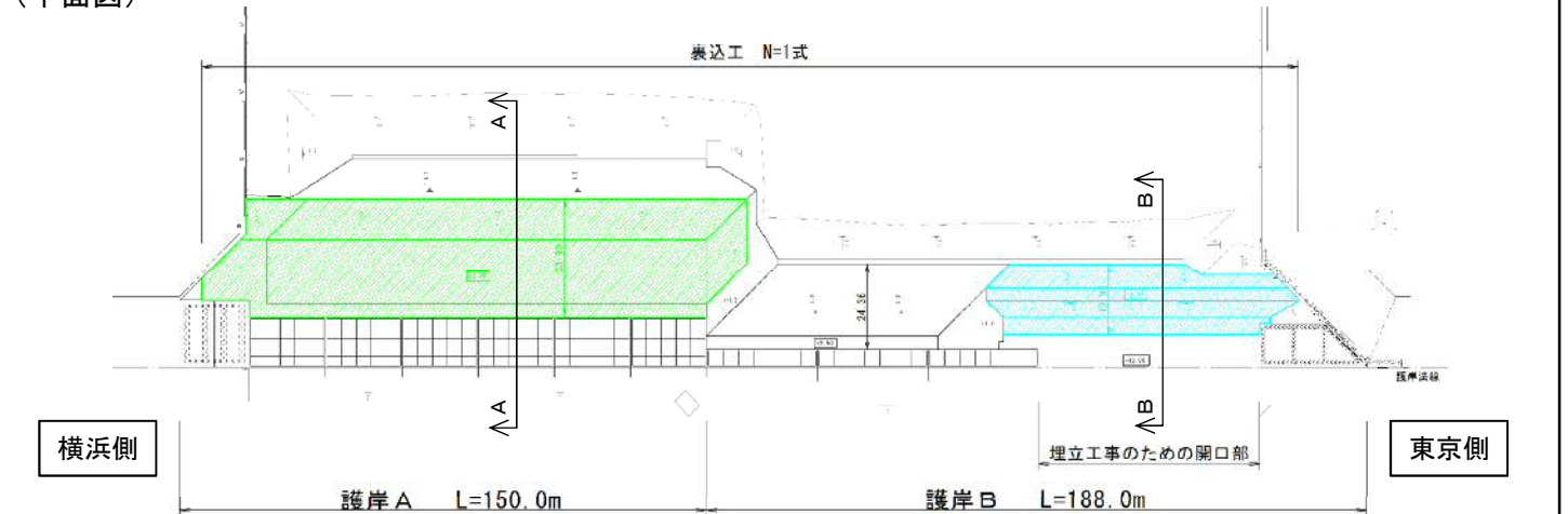
(平面図)
