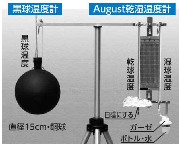
図1 August乾湿温度計と黒球温度計
