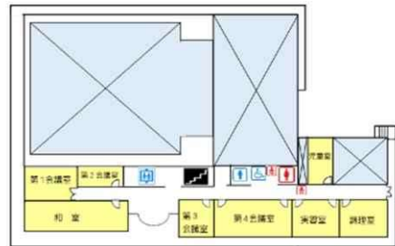
4階平面図
