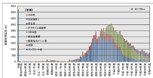
図：管路施設の年度別管理延長(R4末現在)
