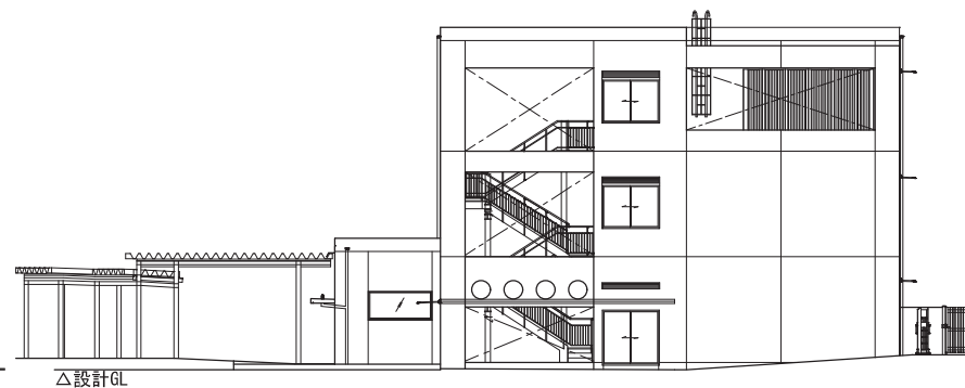
西立面图
