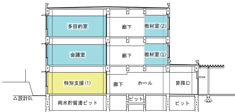
X1-X1' 断面図
