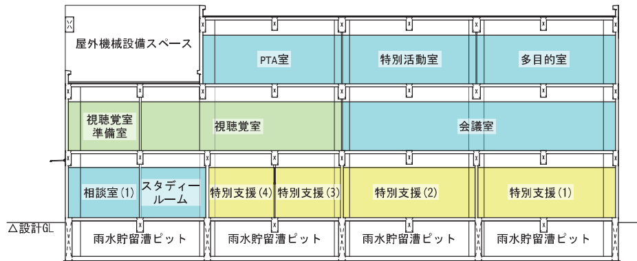
Y-Y' 断面図
