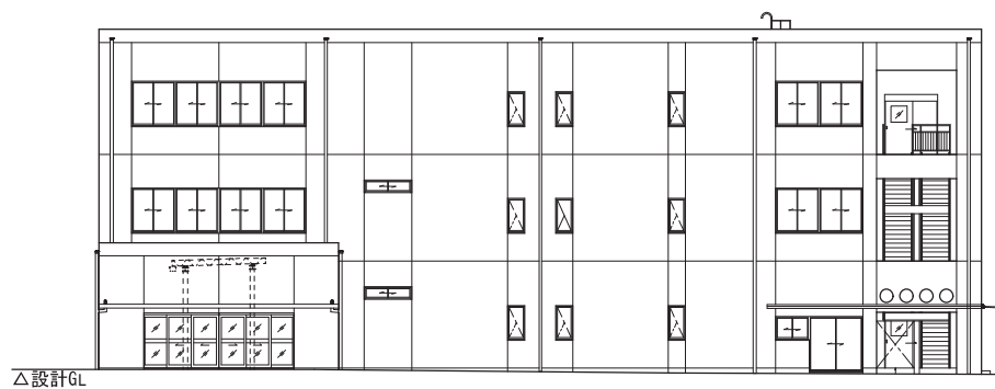
北立面图
