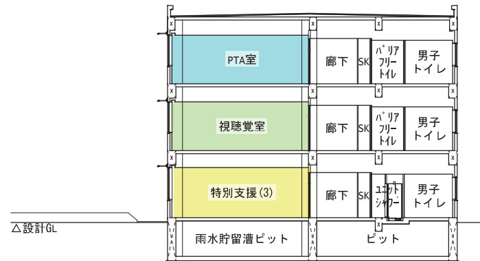
X2-X2' 断面図
