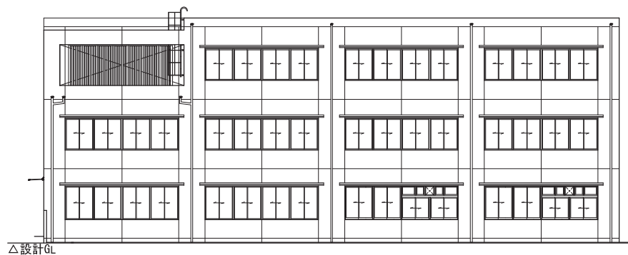
南立面图
