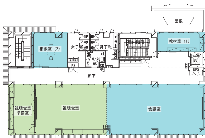
2階平面図
