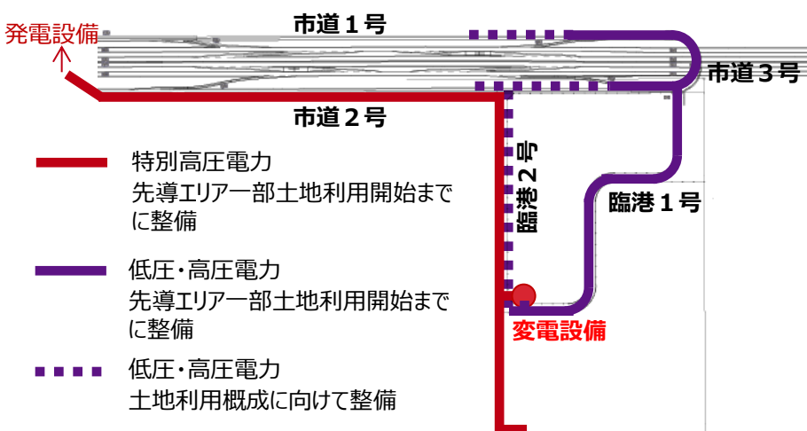
【図21 先導エリア一部土地利用開始時の低圧・高圧、特別高圧電力整備予定箇所（既存発電設備から供給する場合）】
