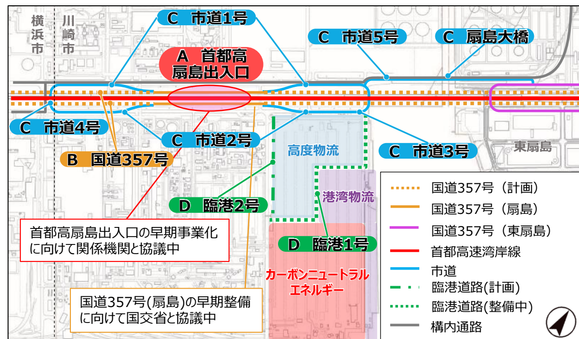
【図4 道路アクセスの取組箇所】
