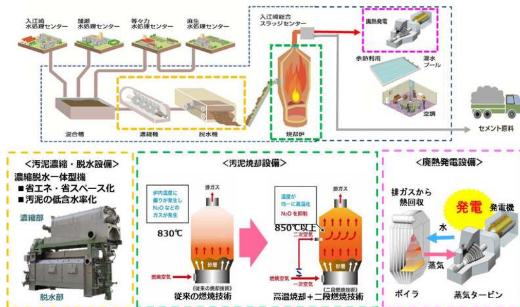
汚泥処理全体フローと汚泥処理技術
