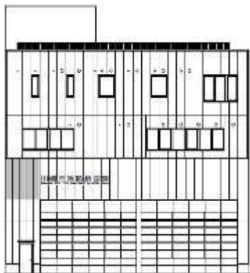
南側立面图
