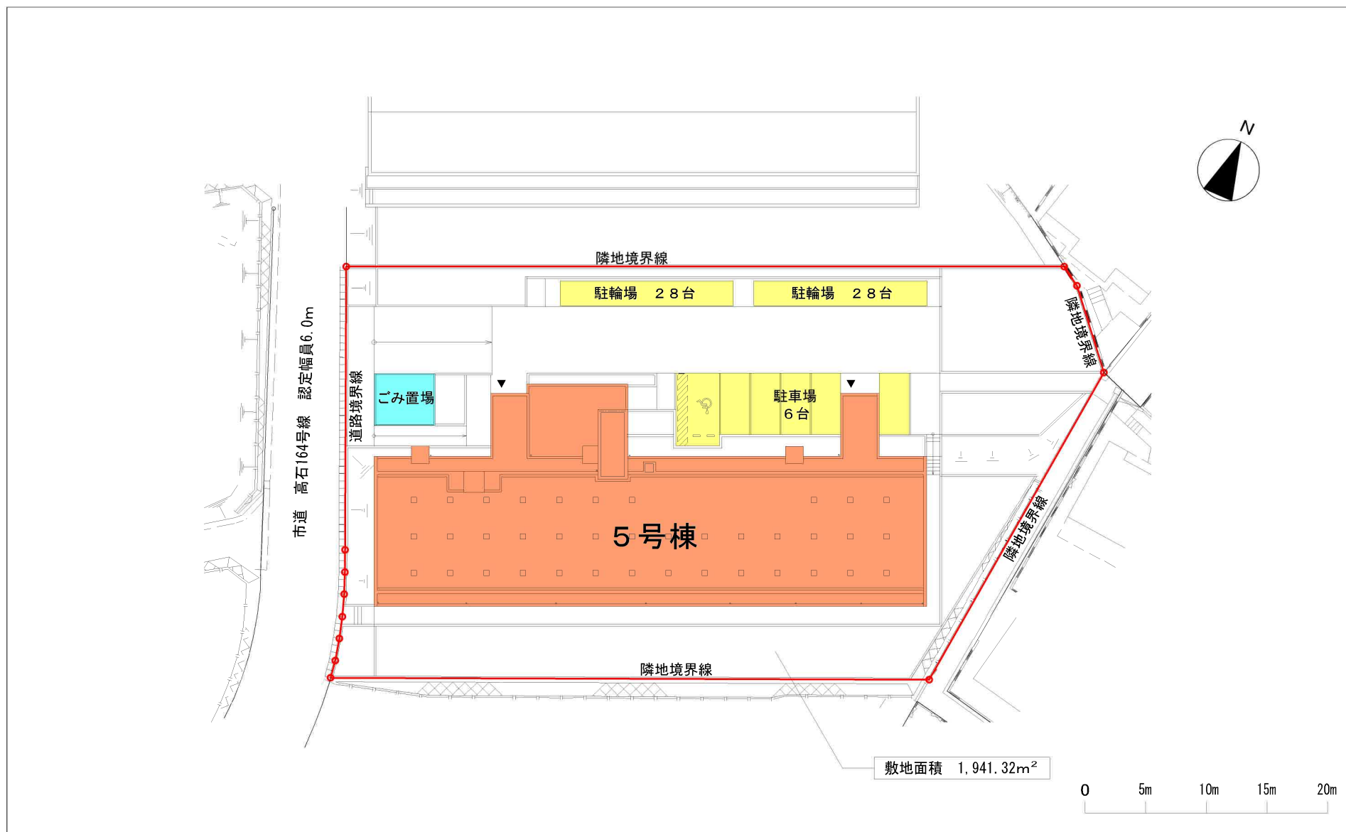
配置図
