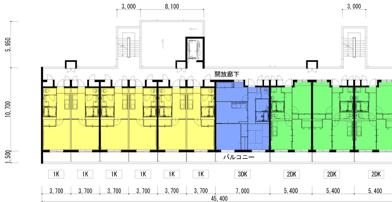
2 階平面図
