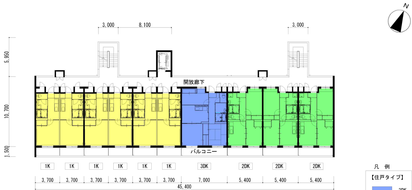
3～5階平面図
