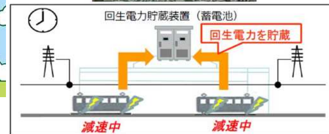
回生電力貯蔵装置（上原駅電所）
