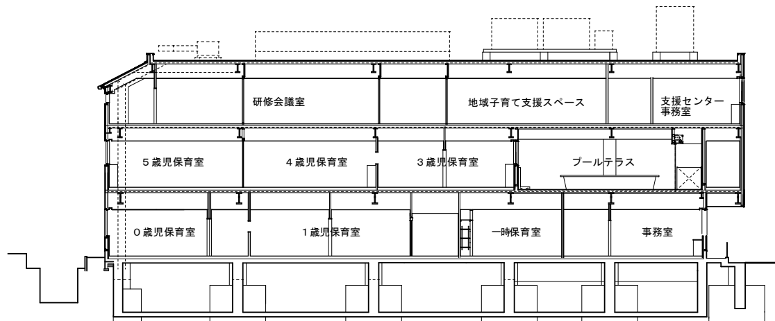
B-B断面図
