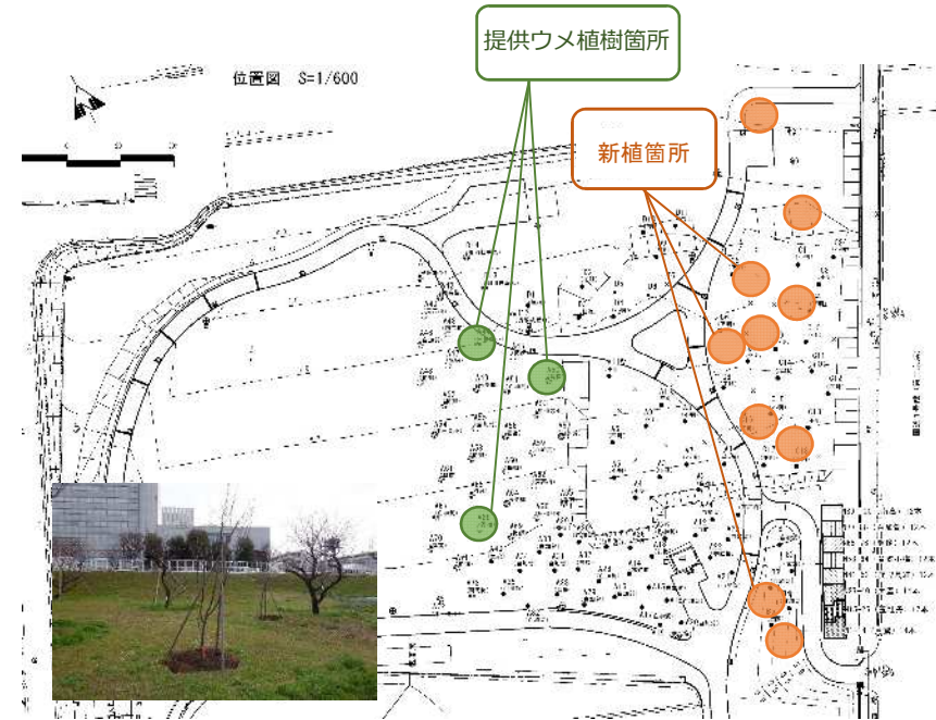
図1 植樹箇所
