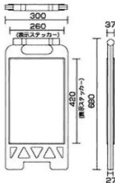
■寸法図 (mm) (折りたたみ時)
