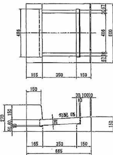
縁塊 (155用)
