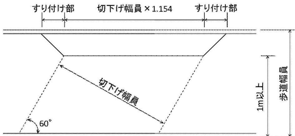
平面図
