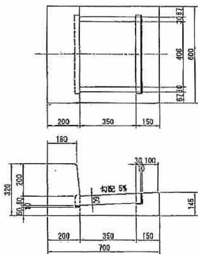
縁塊 (205A用)
