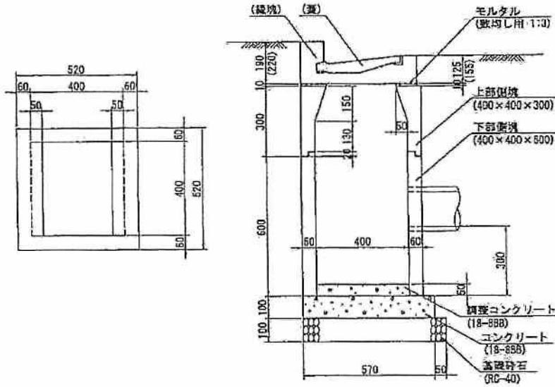
街渠桝縁塊構造図 (参考)
