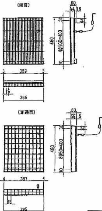
グレーチング蓋
