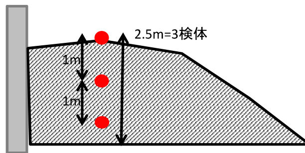
B-B断面
