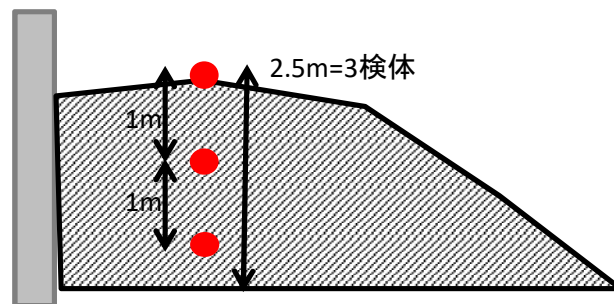
B-B断面
