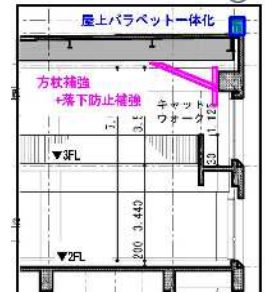
（体育館棟の耐震補強）
