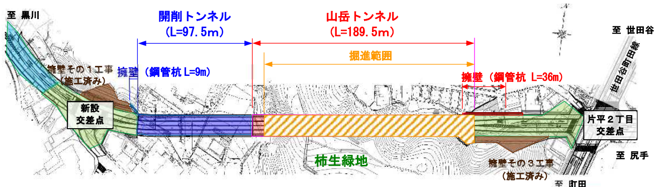
【工事平面図】
