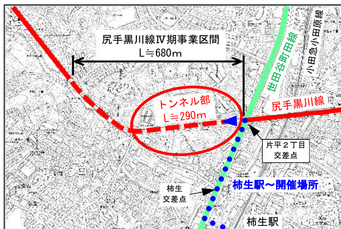
【案内図】
