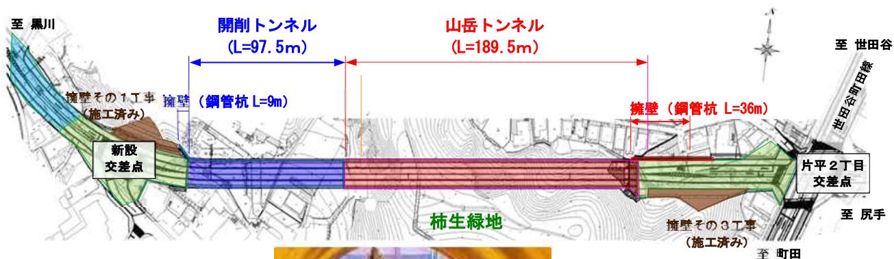
【工事平面図】
