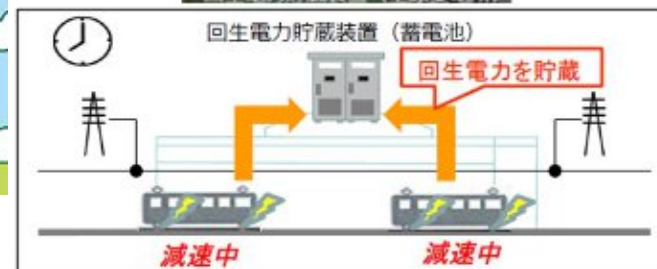
回生電力貯蔵装置 (上原駅電所)
